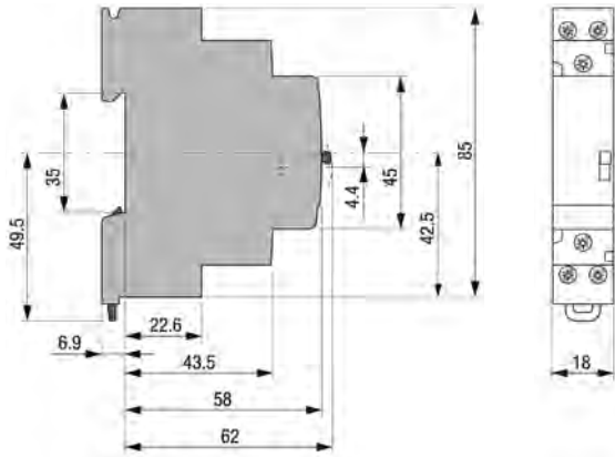
7 E291S Блокировочное реле с циклическим переключением
