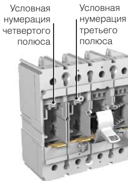
Четырехполюсный выключатель
