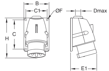
216-432 BS..
