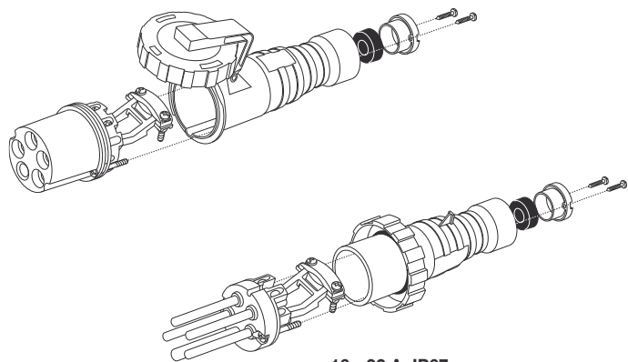
16 - 32 А, IP67
