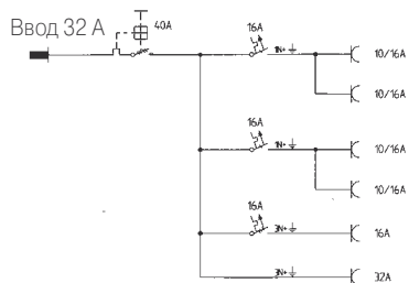
BPC32
