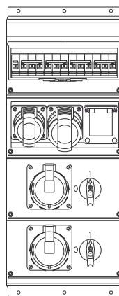
MP32/SW2
