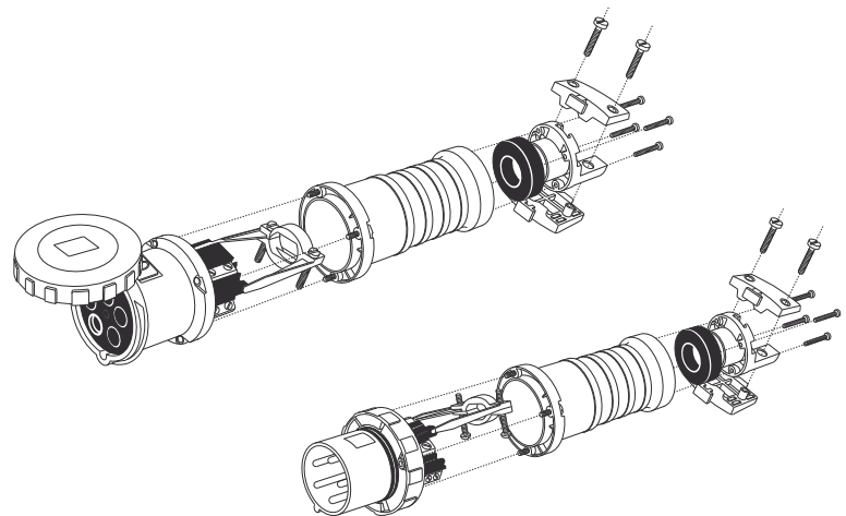
63 - 125 А, IP67
